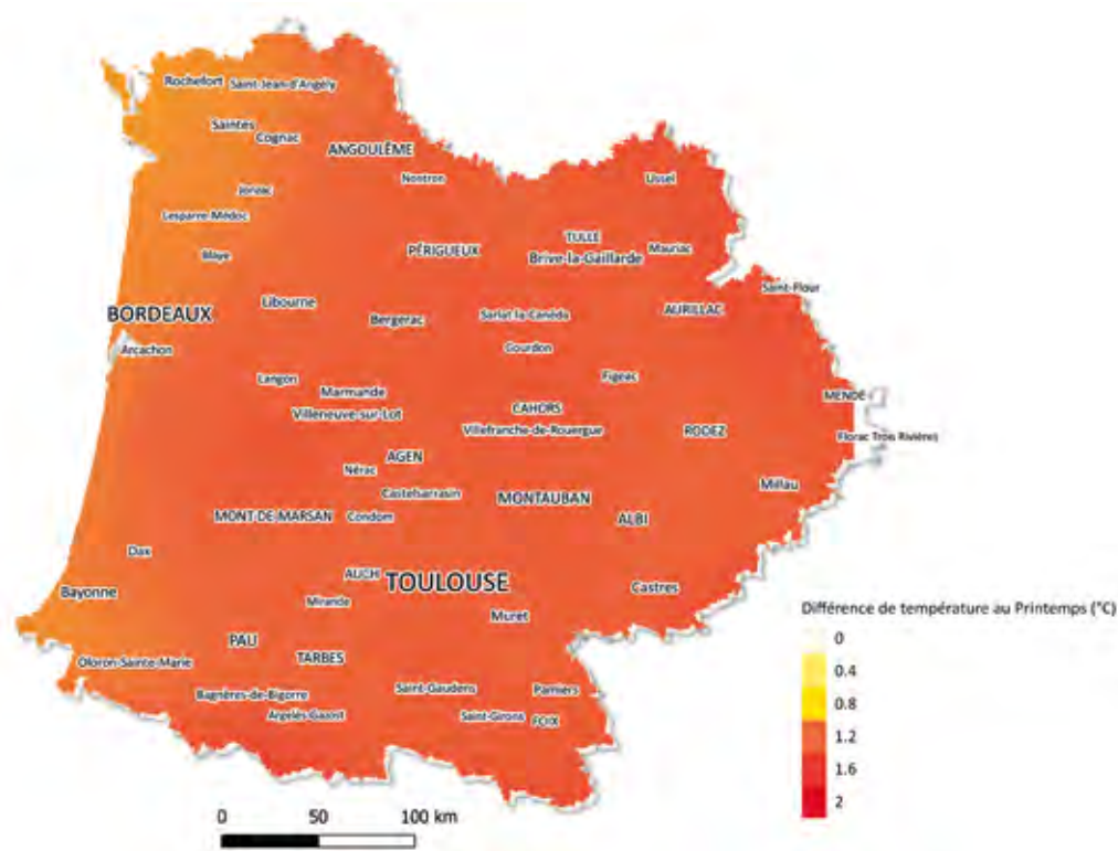
Figure 21 : Anomalie de la température moyenne au printemps - Scénario médian (RCP 45) - horizon proche (2021-2050) par rapport à la période référence 1950-2005 (DRIAS les futurs du climat)
